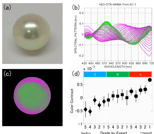
図1：真珠の光学特性と熟練者評定の関係。(a)真珠像、(b)真珠に見られる干渉色スペクトルの偏角依存性、(c)干渉色の可視化結果、(d)熟練者評定（横軸）と干渉色の空間コントラスト（縦軸）との関係。
