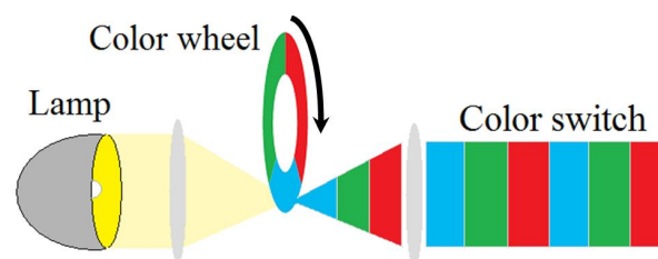
図：DLPのカラースイッチ機能に基づく光源色の変化を利用
