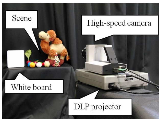
図1：動的なシーンに適用可能な分光計測技術の開発を進めました。
