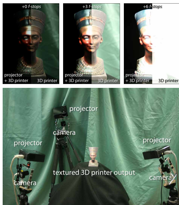
図1：カラー3次元プリンタから出力された模型に複数台のプロジェクタを使って映像を投影して、文化財を高いコントラストで再現します（上段：映像を投影した場合としない場合でのコントラストを比較するため異なる露光時間で撮影した画像、下段：実験風景）。
