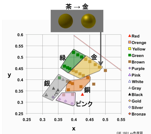
図: 光沢感変化に伴う金銀銅色の色度範囲の変化。光沢レベル最小の条件でのカテゴリカルカラーネーミングの結果に対して、光沢レベル最大の条件で金銀銅色と評価された色度点が囲み線で示されています。
